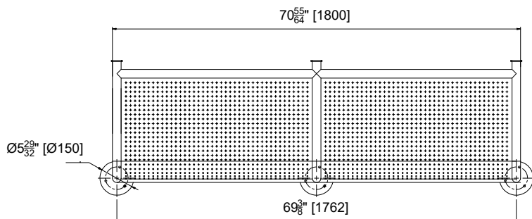
MODEL US-SWM-B Plan
